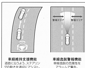
LKAS作動イメージ
