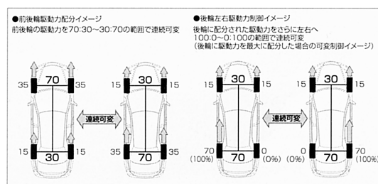
駆動力可変範囲
