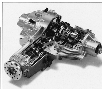
SH-AWDリアドライブユニット・カットモデル
