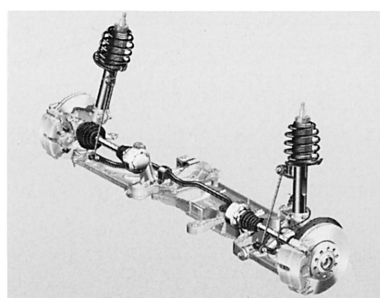
進化させたマクファーソンストラット式 フロントサスペンション
