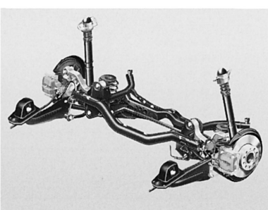
新開発の4リンク式リヤサスペンション
