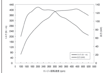
■ SKYACTIV-D 2.2エンジン性能曲線
